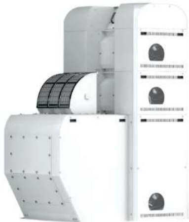
6-ти вальцевая дробилка Maltomat™ III MDBA для пивоварен 500 гкл
